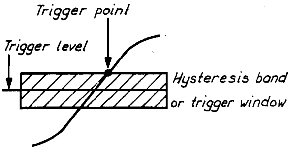
Fig. VI-2. Triggering
