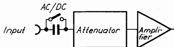
Fig. VI-1. AC/DC coupling
